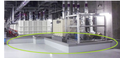
防液堤 地下・公共水域への流出防止
